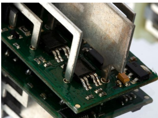
Detailansicht mechanisches Relais (oben) vs. intelligente Halbleiter im Hitachi Produkt (unten)
