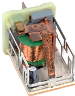
Links: Glühzeitrelais eines OE-Anbieters Rechts: Hitachi Produkt 250 2183
